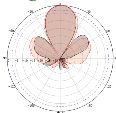
Feldschemata/radiation patterns
